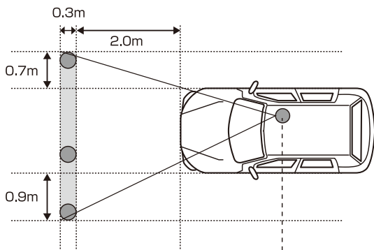
上面図
